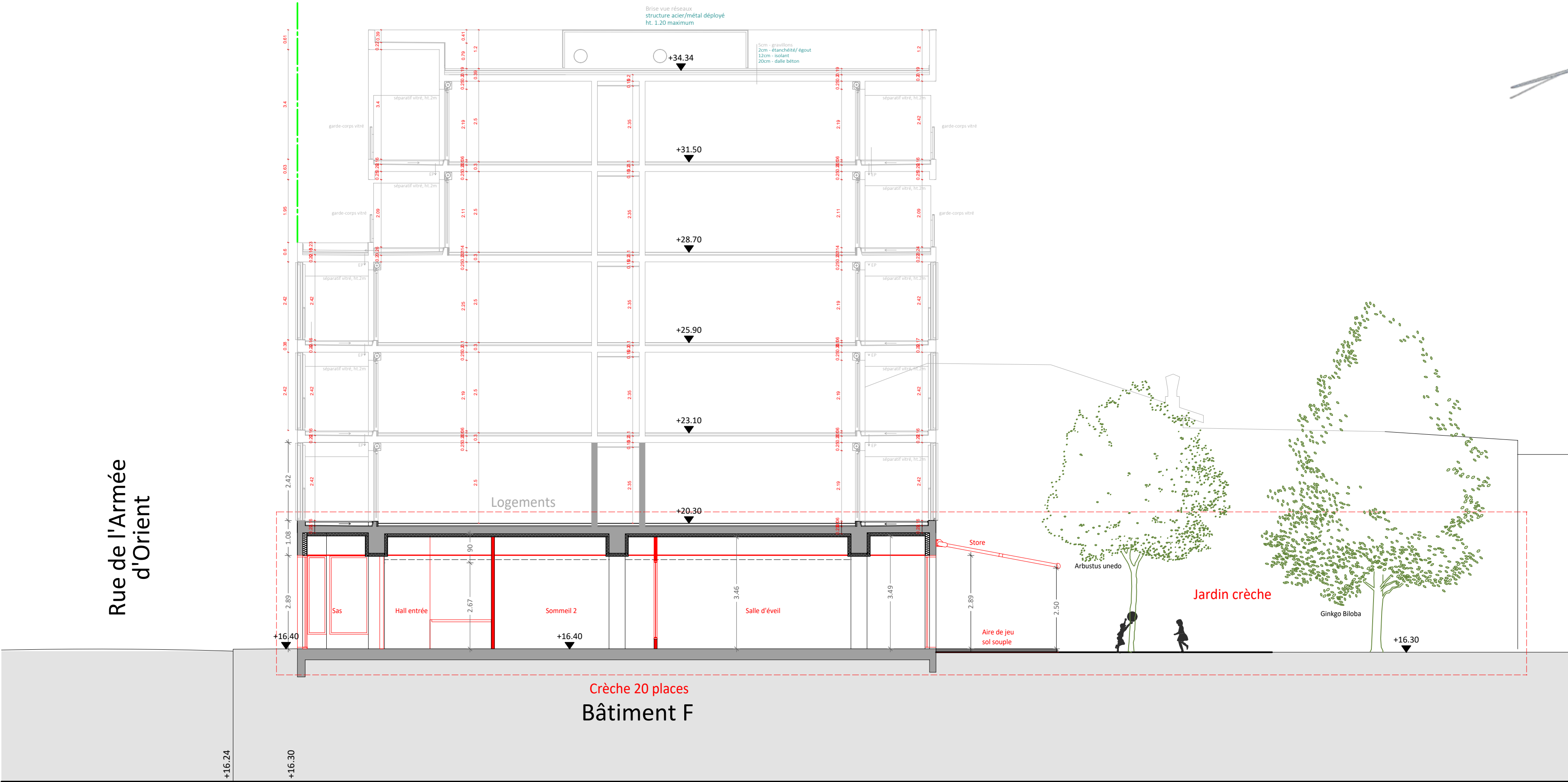
COUPE LONGITUDINALE - BAT F Coupe modifiée pour le changement de destination d'un local artisanal en crèche de 20 places
